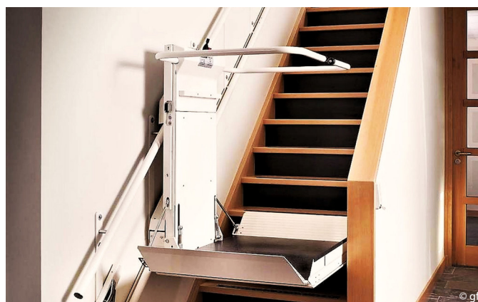
Plattformlift innen
